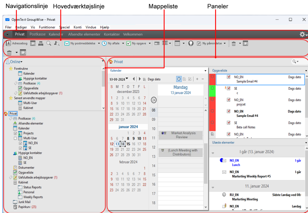
Figur 8-1 Hovedvinduet
