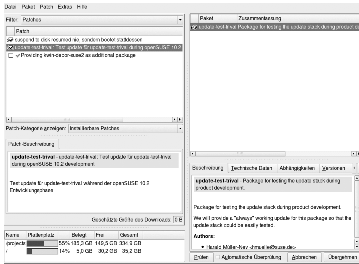
Abbildung 1.1 YaST-Online-Update
