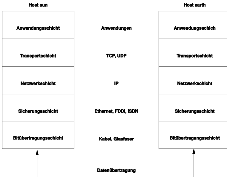
Abbildung 19.1 Vereinfachtes Schichtmodell für TCP/IP
