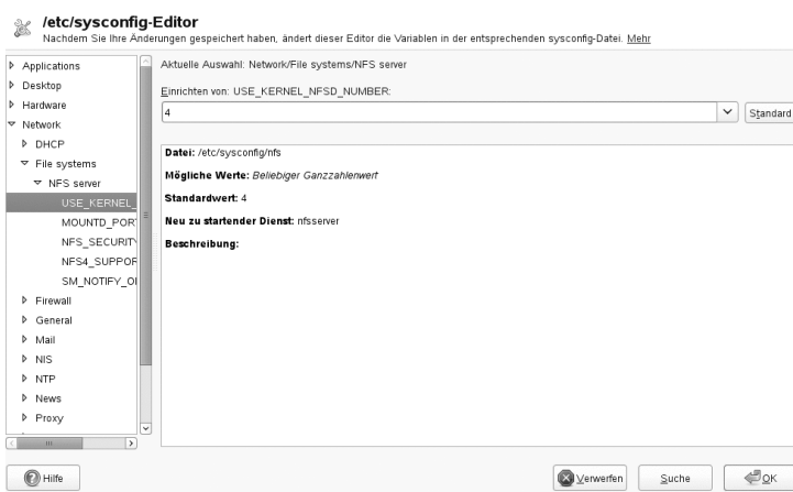
Abbildung 9.2 Systemkonfiguration mithilfe des sysconfig-Editors
