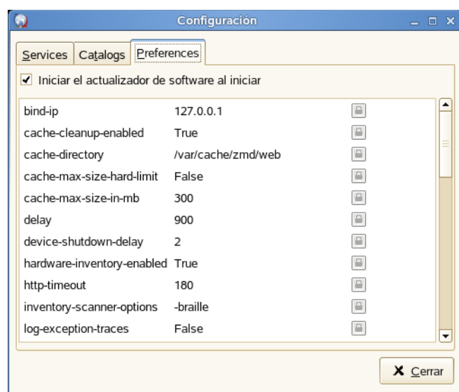
Figura 1-23 Cuadro de diálogo de configuración de las preferencias del actualizador de software
