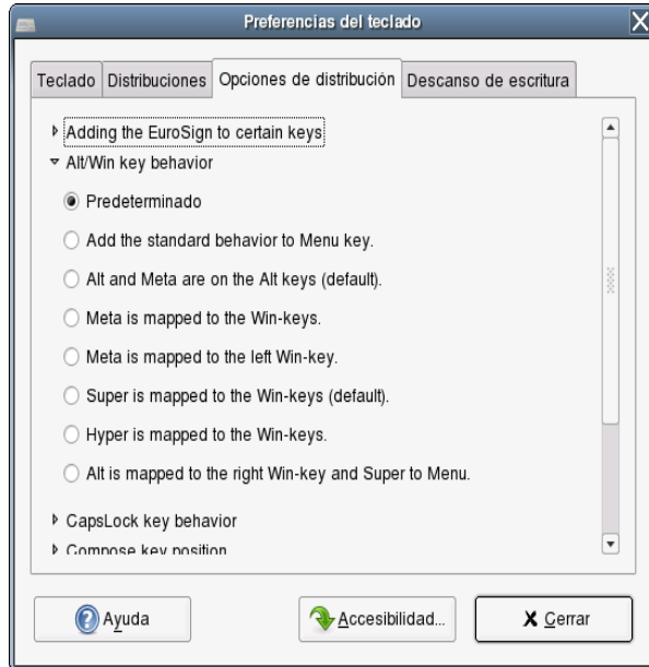
Figura 2-4 Cuadro de diálogo de preferencias del teclado: pestaña Opciones de distribución
