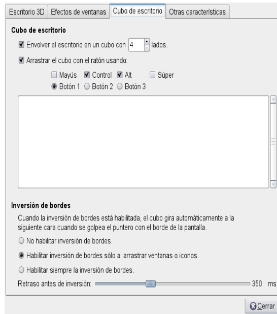
Figura 2-14 Pestaña Cubo de escritorio
