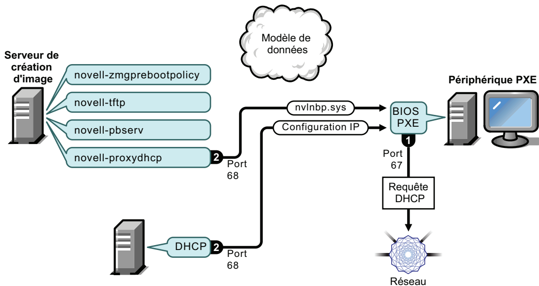
Figure 25-1 Configuration DHCP sur des serveurs séparés
