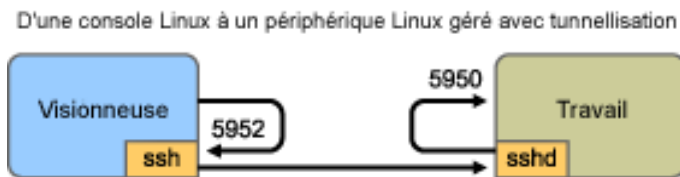
Figure I-1 Console Linux vers périphérique géré par Linux avec tunnel
