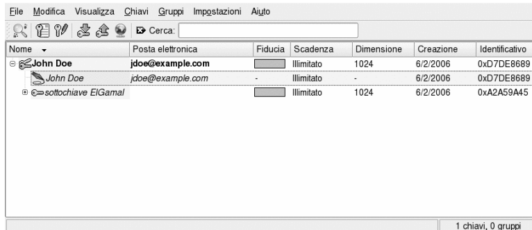
Figura 10.2 Gestione chiavi
