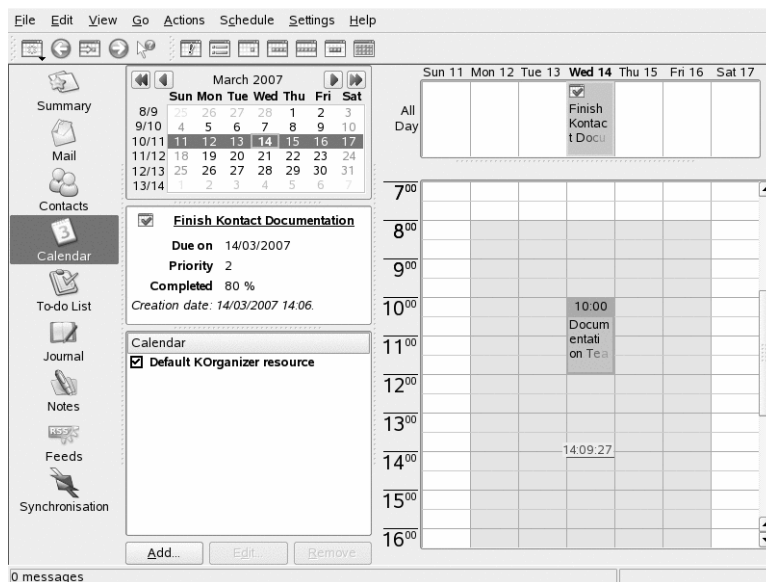
Figur 4.4 Kontakt-kalenderen
