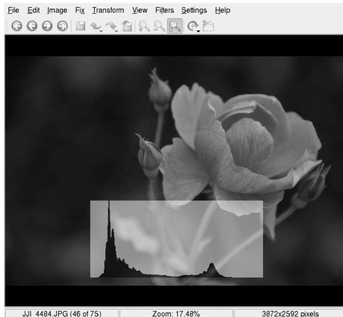
Figur 19.5 Kontrollere histogrammet
