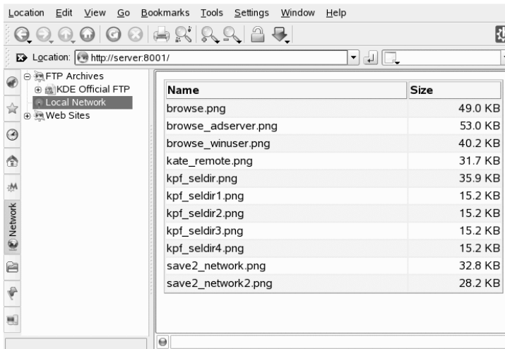
Figur 9.15 Publisert innhold
