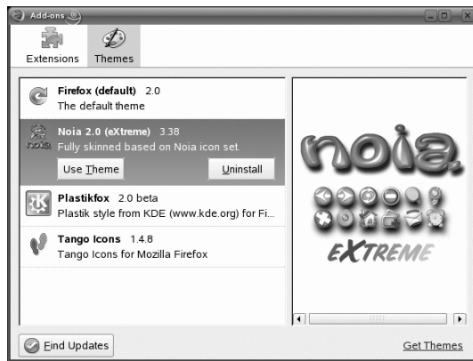
Figur 15.4 Installere Firefox-temaer
