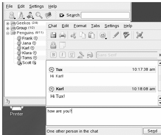
Figur 7.1 Direktemeldingsvindu
