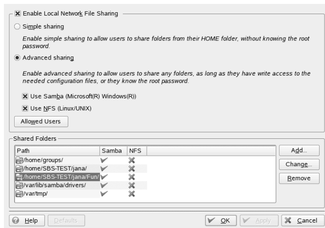
Figur 9.2 Aktivere fildeling
