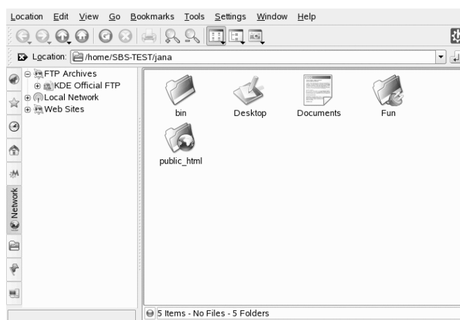
Figur 9.4 Delt mappe
