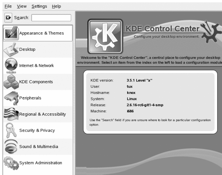
Figur 2.1 KDE kontrollsenter
