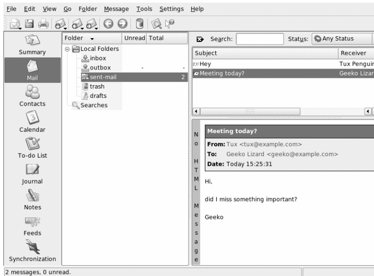
Figur 4.2 Kontakt Mail-komponenten
