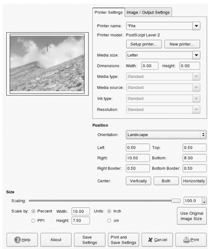
Figur 18.3 Utskriftsdialogboksen
