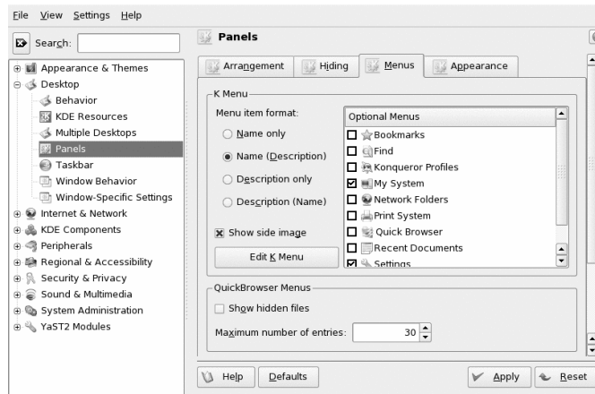
Figur 2.3 Redigere hovedmenyen
