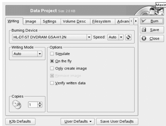
Figur 21.2 Tilpasse brenneprosessen
