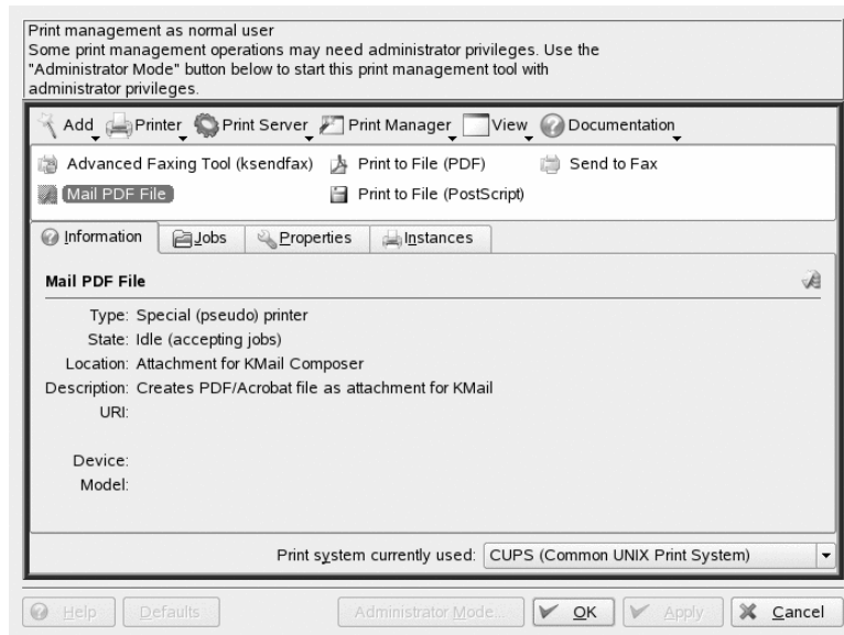
Figur 12.1 Utskriftsbehandler
