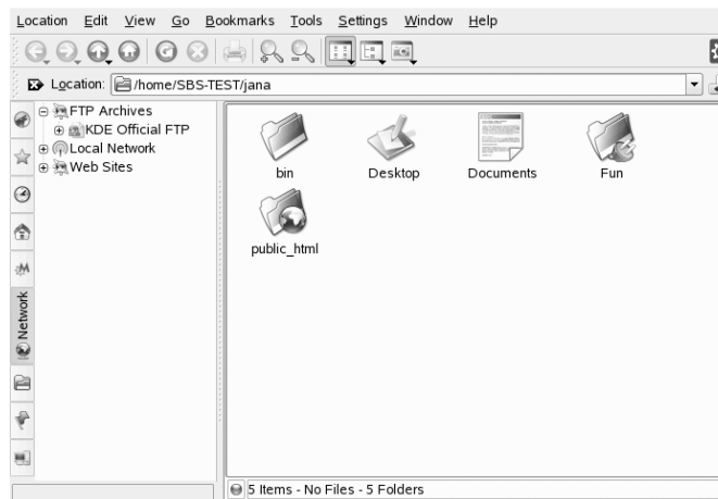
Figur 9.4 Delad katalog
