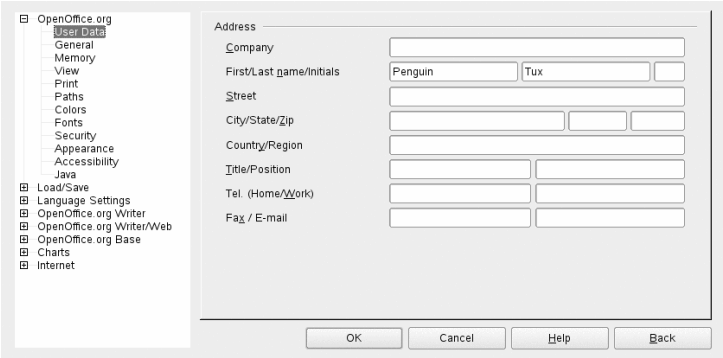
Figur 3.1 Alternativfönstret
