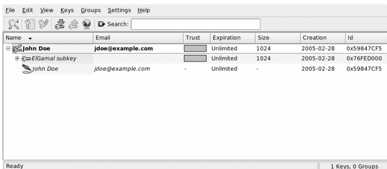
Figur 10.2 Nyckelhanteraren
