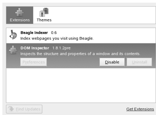
Figur 15.3 Installera Firefox-tillägg
