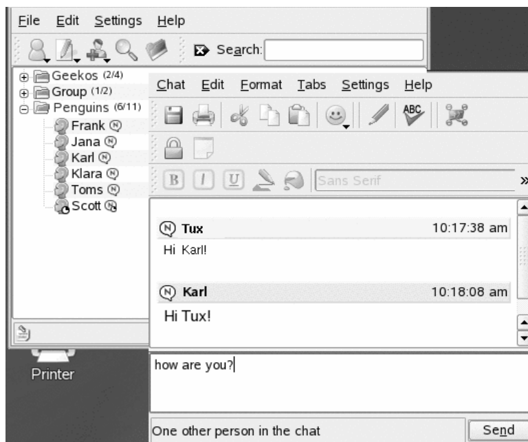
Figur 7.3 Chatisfönster
