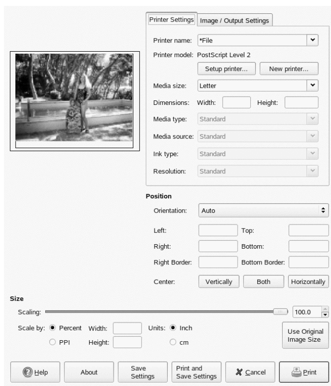
Figur 18.3 Utskriftsdialogrutan
