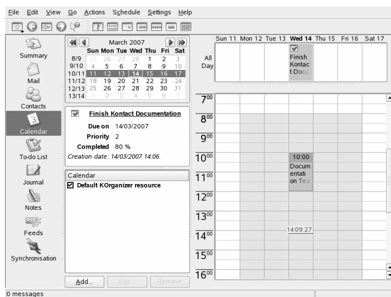
Figur 4.4 Kontakt-kalendern
