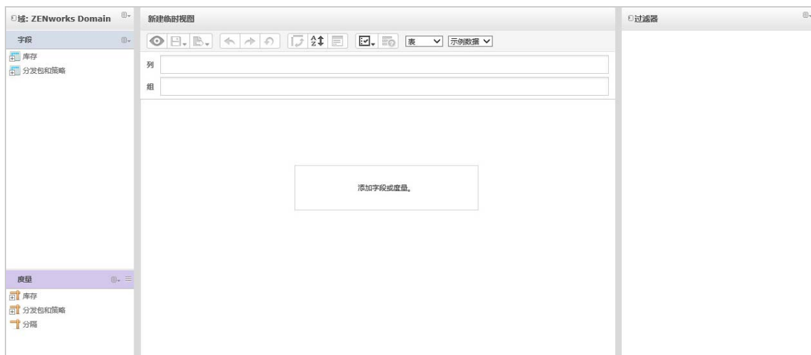
图2-1 专用编辑器
