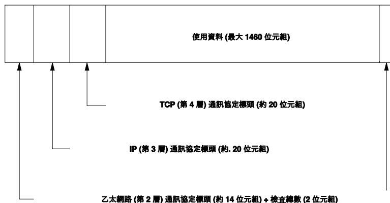
圖形 19.2 TCP/IP 乙太網路封包
