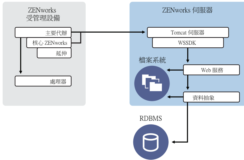
圖 2-3 ZENworks 10 用戶端- 伺服器結構
