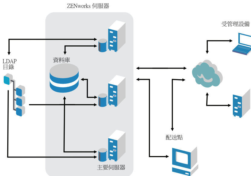
圖 2-4 ZENworks 10 的結構
