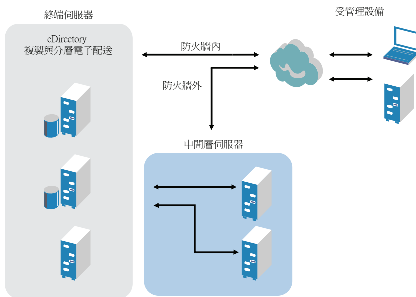
圖 2-1 ZENworks Desktop Management 的結構
